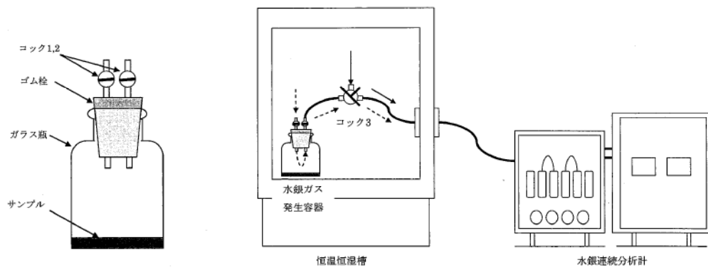
図2-2 a) 水銀ガス発生容器
