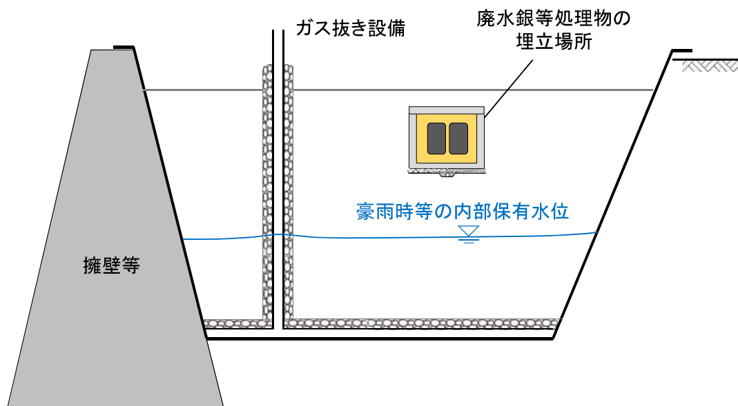
図 3.7.2 廃水銀等処理物の埋立場所の例
